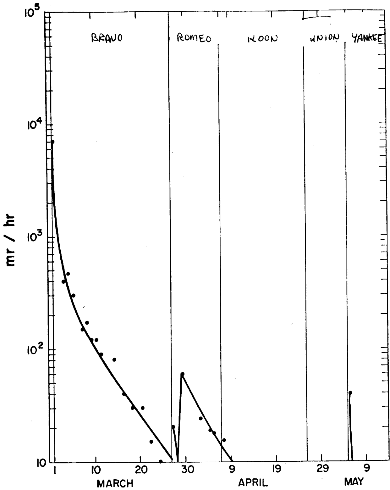
Fig. 4.8—Fall-out record, Aitukijl.
